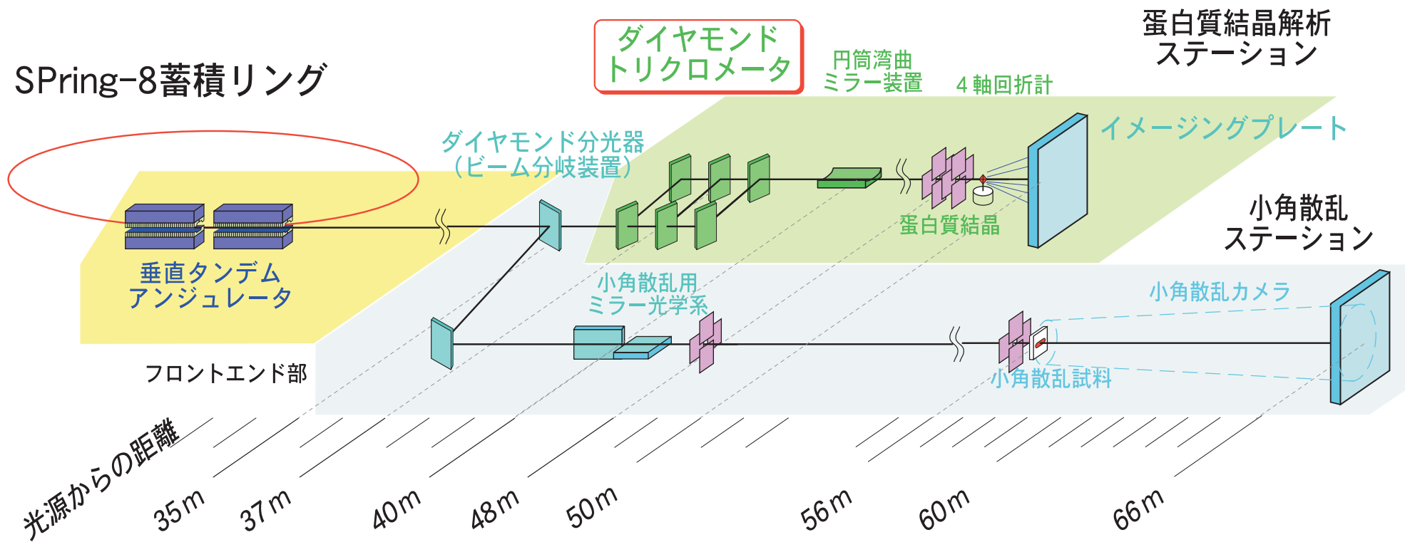
理研ビームライン I (BL45XU)の全体像
