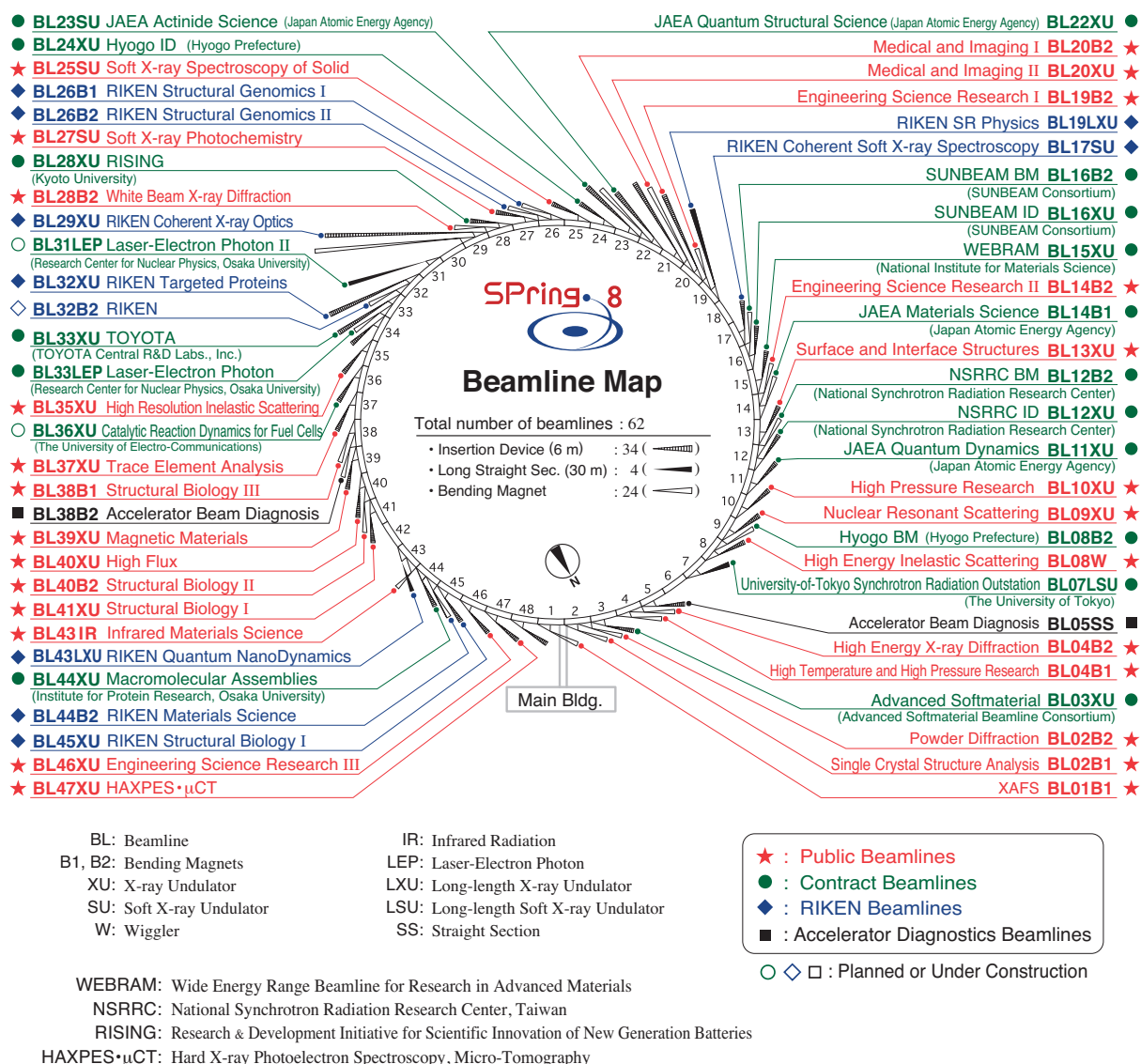
Fig. 2. Beamline map.
