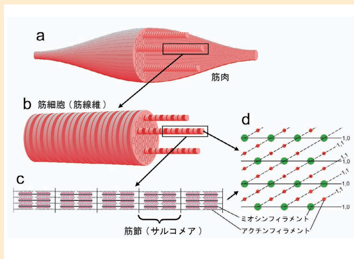
図1. 脊椎動物の骨格筋(横紋筋)の構造。a. 全筋。多数の筋細胞(筋繊維)が集まってできている。b. 筋細胞。直径50~100マイクロメートル。直径1~2マイクロメートルの筋原繊維が多数集まってできている。c. 筋原繊維の拡大図。長さ2~2.5マイクロメートルの筋節(サルコメア)が多数直列に並んでいる。この中で収縮タンパクミオシンとアクチンのフィラメントが六角格子の形に並んでいる(d)。1個の筋節中では格子の向きは揃っている(単結晶)。格子の中には多数の線で示したように「格子面」とよばれる面があり(示した以外のものもたくさんある)、それぞれに1,0とか1,1などの名前がついている。
