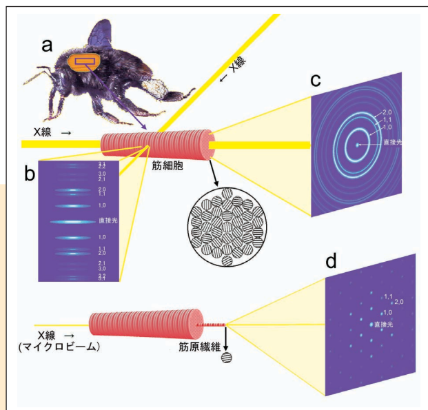
図2. マルハナバチ飛翔筋の筋細胞からX線回折像を記録する方法。a、マルハナバチ。b、いままでの方法によるX線回折像記録（X線を筋細胞の軸と直角にあてる）。筋細胞に多数含まれる筋原繊維中の六角格子の向きはランダムなので全ての格子面からの反射が重なってしまう。c、エンドオン回折像記録。X線を筋細胞の軸に沿って照射する。この場合も、X線の径が大きい場合は多数の筋原繊維にX線があたるため、回折像は同心円状になり、反射はやはり重なってしまう。d、X線マイクロビームにより筋原繊維1本からエンドオン回折像を記録した場合。X線の中に1本の六角格子しか含まれないので、それぞれの格子面からの反射がスポットとして分離して記録される。
