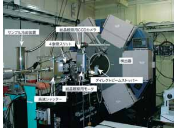
図2 DIP6040を利用したデータ収集系
