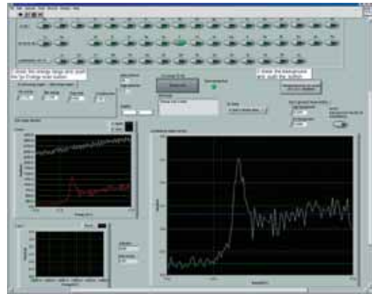
図3 CHOOCH++の1画面
