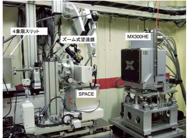
図2 データ収集系
