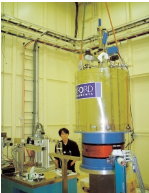
強磁場極低温X線磁気散乱実験用15T超伝導マグネット。27mアンジュレータを光源とするBL19LXUの実験ハッチ4に設置された。
