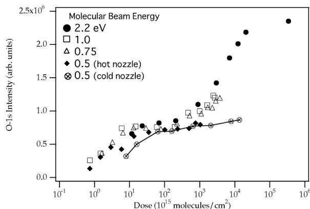
図 1 Cu(511) 表面の超熱酸素分子線による解離吸着曲線—入射エネルギー依存性—
