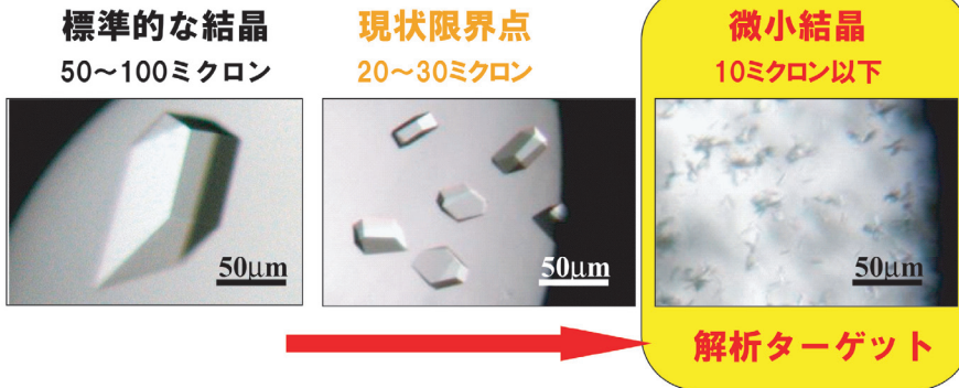
図1 本ビームラインで解析可能にするタンパク質結晶サイズ
