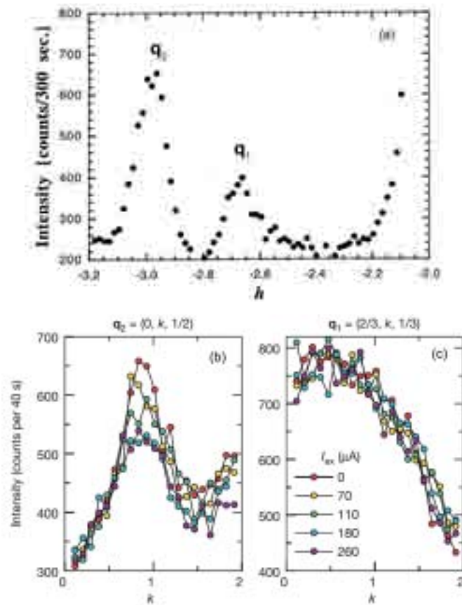
図2 有機サイリスタの低温X線散漫散乱。(a)20 Kにおける散漫散乱。 q_1 、 q_2 で指定される2つの電荷秩序からの散漫散乱が同時に観測されている。横軸は、 a^*c^* 平面 (BEDT-TTF層の面内方向)で2つの散漫散乱を結ぶ方向の逆格子位置を表す。(b) q_2 散漫散乱の依存性。(c) q_1 散漫散乱の電流依存性。(b)(c)の横軸は、 b^* 軸 (BEDT-TTF層の面間方向)の逆格子位置を表す。 q_2 が面間方向にもピークを持つものに対して、 q_1 は面間方向にほぼフラットな強度を持つ。このことは、前者が擬3次元的な短距離秩序、後者が2次元的な短距離秩序を示している。
